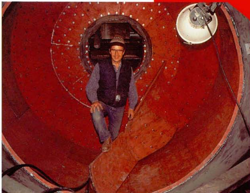
Kvarninfodring med Linard 60 "strapbak"
